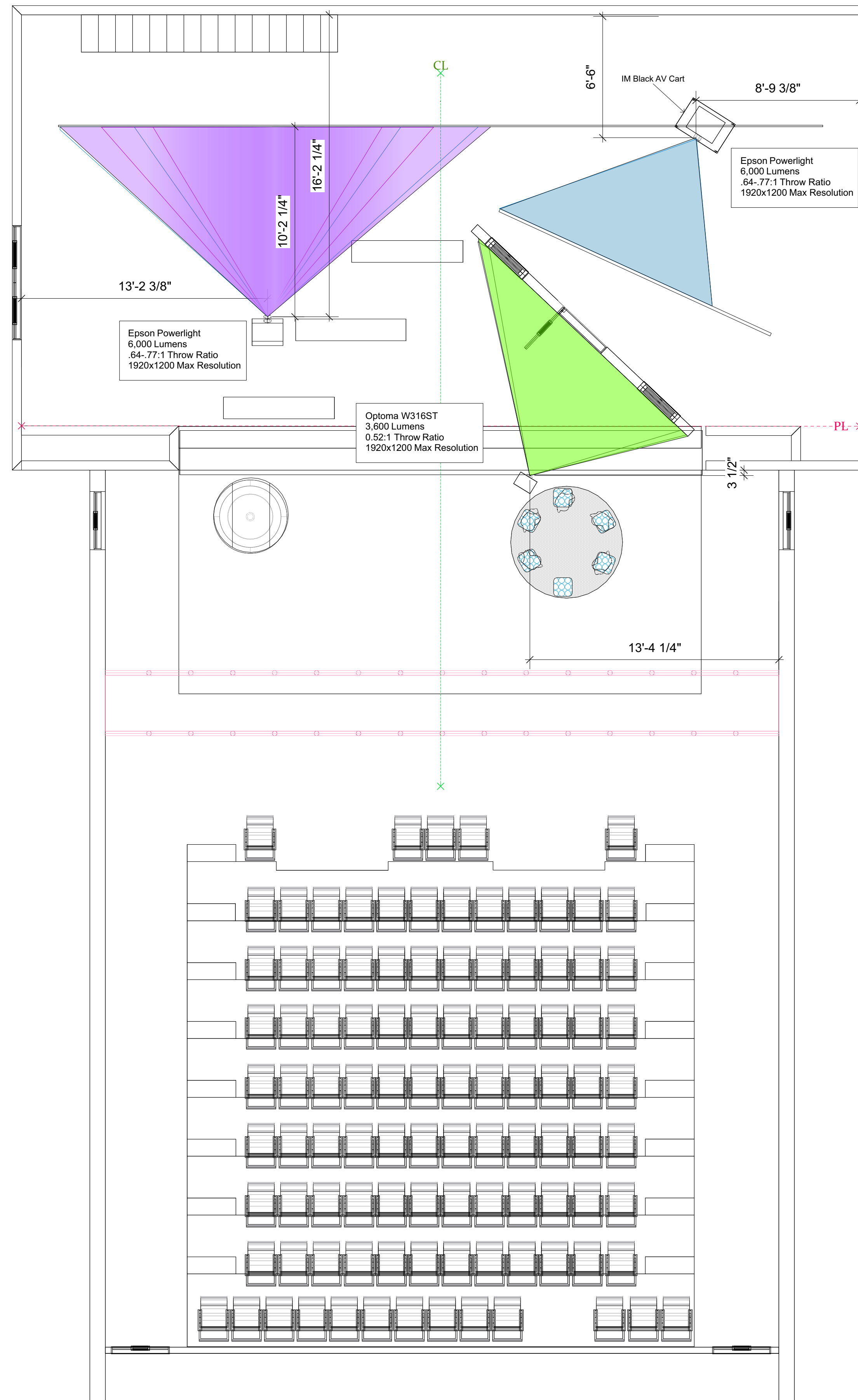
2 Plan Top Scale: 1/4" = 1'-0"
